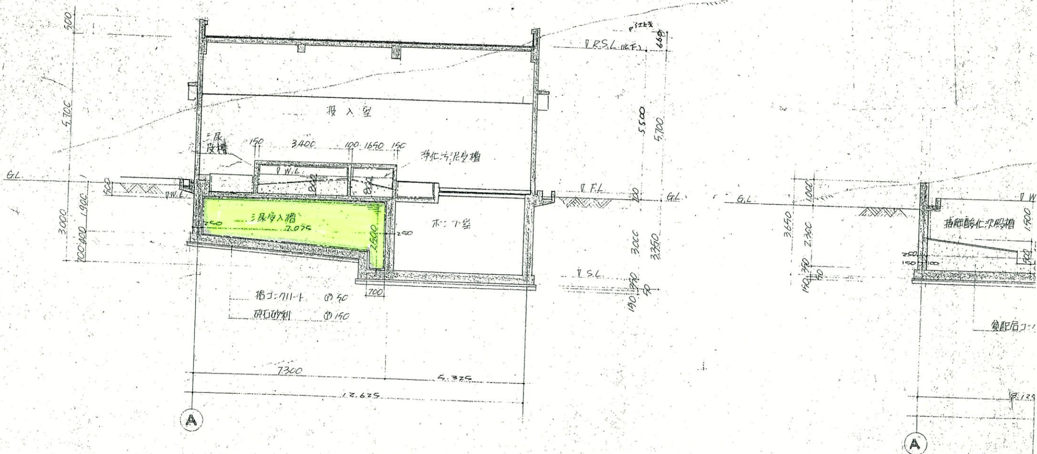
D—D 断面図
