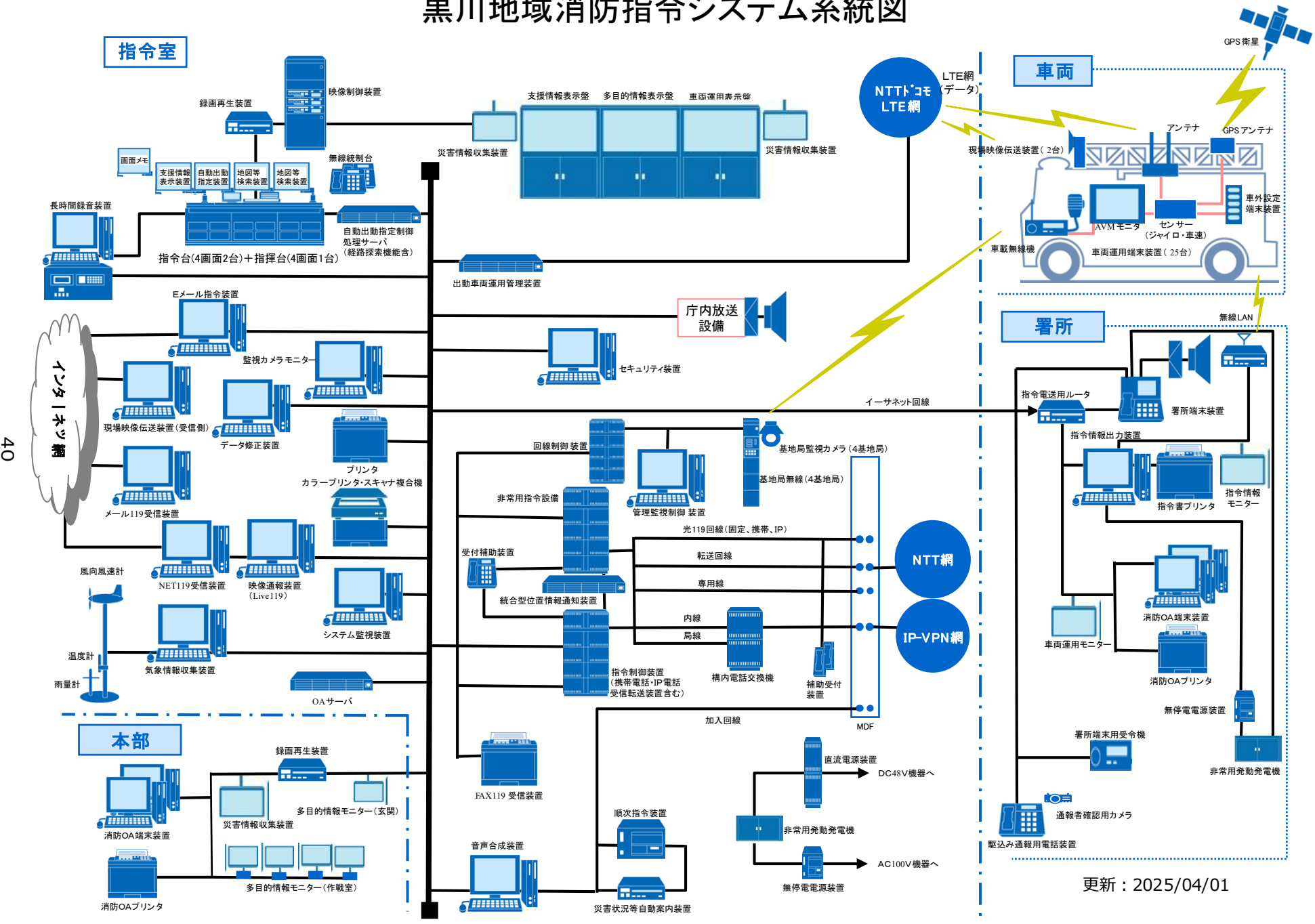
機器構成図（システム系統図）
