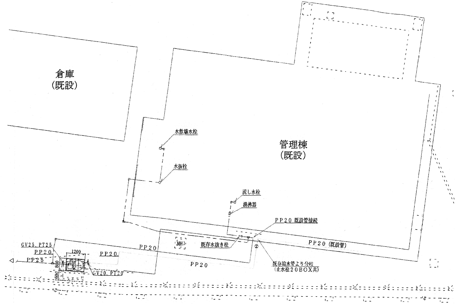
既存給水管接続図 S=1/100
