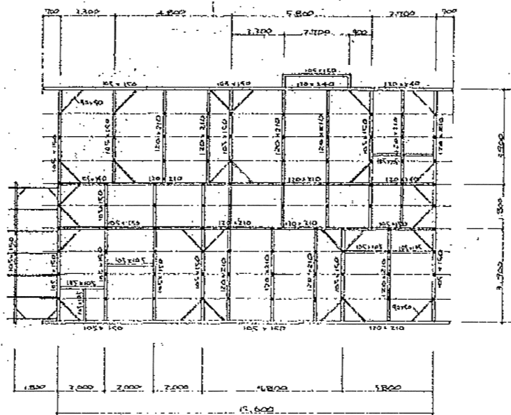
小屋伏図 1/100
