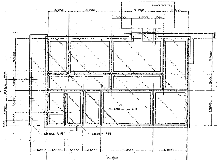
基礎伏図 1/100
